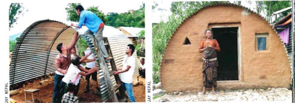
Ideato dall'Istituto di ingegneria di Patan, lo shelter (sopra) è una struttura per 5-6 persone capace di resistere a forti piogge. Formato da 8 pannelli di alluminio ondulato sovrapposti e chiuso con mattoni o legno, costa circa 150 euro. Così Jay Nepal ha dato riparo a oltre 2mila abitanti.
