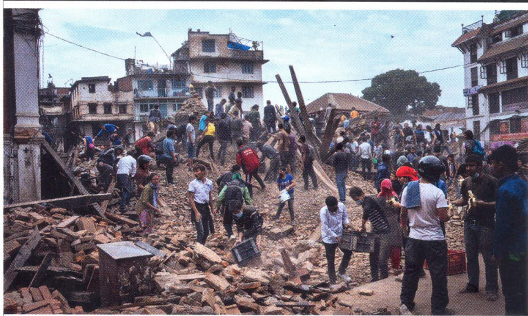
Le macerie di Kathmandu, devastata da un terremoto il 25 aprile. Dopo nove giorni sono stati estratti ancora dei superstiti. Il sistema sanitario è al collasso e ci vorranno anni per ricostruire il Nepal.
